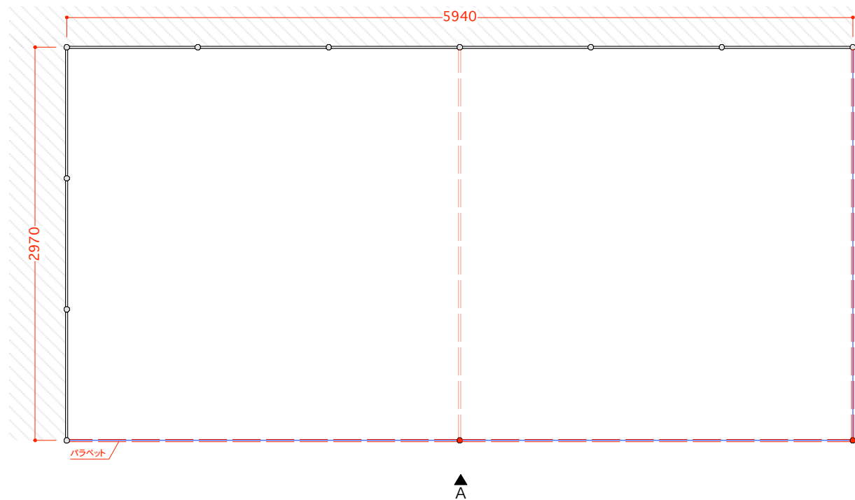
■ layout 2小間L字右側オープン(W5940xD2970xH2700) 基礎壁システムパネル
